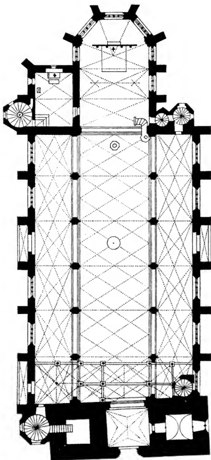
2. Grundriß.
