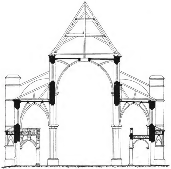
5. Querschnitt.
