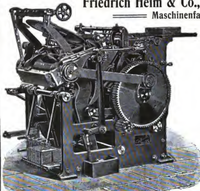
Sicherheits-Tiegeldruck-Schnellpresse „Der Falke“, Patent Waite
