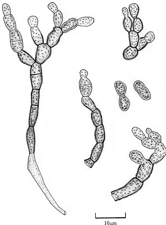
Fig. 10 Cladosporium arthoniae (hb. Christiansen 570—holotype).
