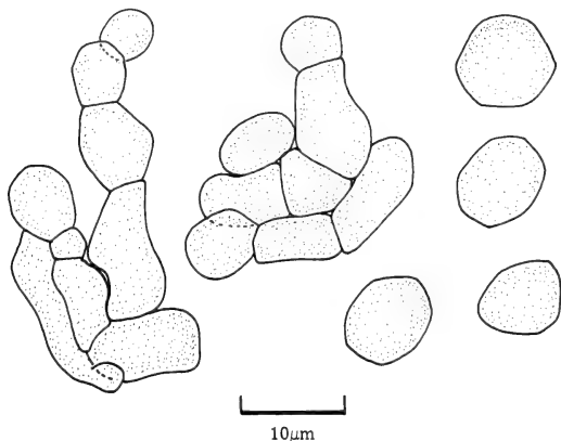
Fig. 25 Illosporium corallinum (K—istotype).
