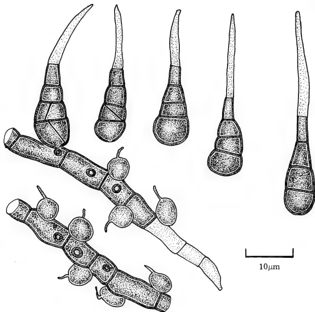
Fig. 12 Dictyophrynella bignoniacearum (URM 28007—holotype).
