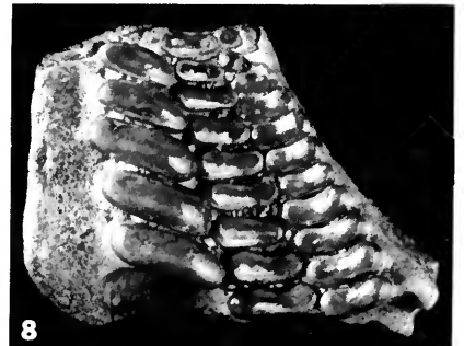
Figs 3–8 Splenials of P. maliensis sp. nov., all except Fig. 3 \times 1 . Fig. 3, holotype BMNH P.61048, \times 2 . Fig. 4, paratype BMNH P.60631. Fig. 5, paratype BMNH P.60625. Fig. 6, paratype TGE 60L. Fig. 7, paratype BMNH P.60628. Fig. 8, paratype BMNH P.60920.
