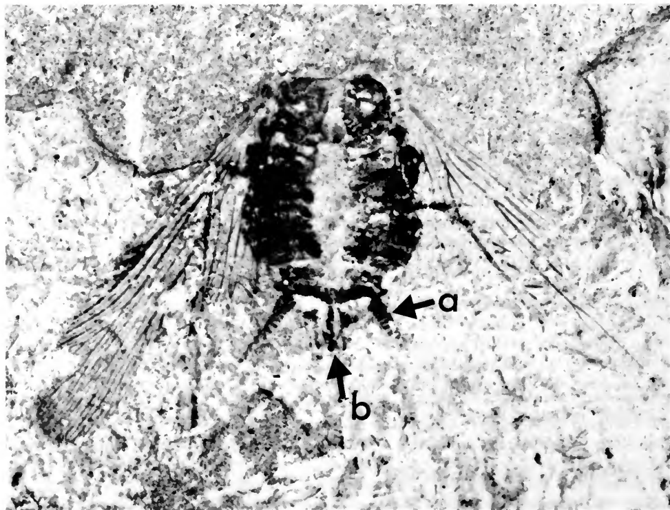
Fig. 7 Artitocoblatta hispanica sp. nov. (cockroach). Holotype. In.59505, \times 13 . (a - cercus; b - ovipositor).
