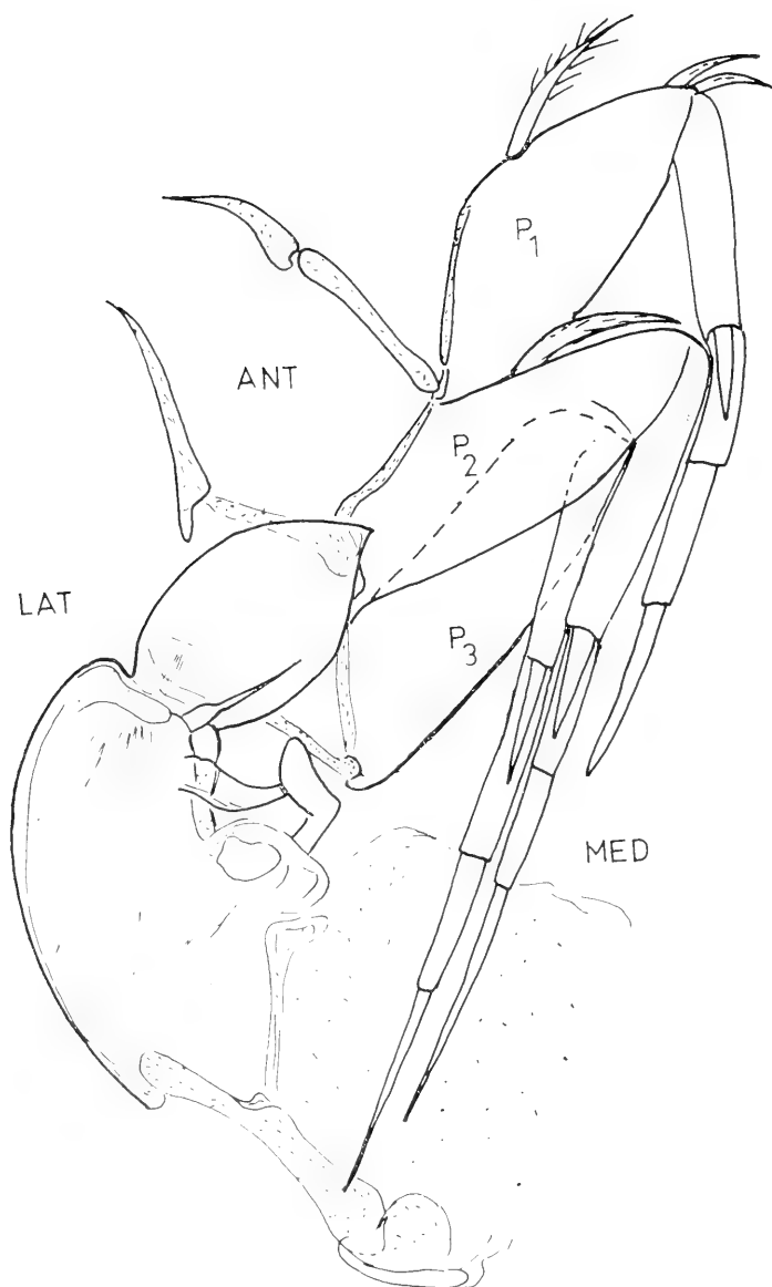
Text-fig. 6. Elpidium , n. sp. B, mâle. L'organe copulateur droit en position normale sur la partie postero-ventrale du corps (P 1 — P 3 — thoracopodes. LAT — côté latéral. MED — côté médial; ANT — antérieur).
