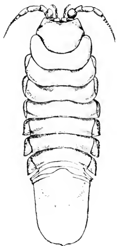
FIG. 402.—PENTIDOTEA WOSNESENSKII. MALE.
