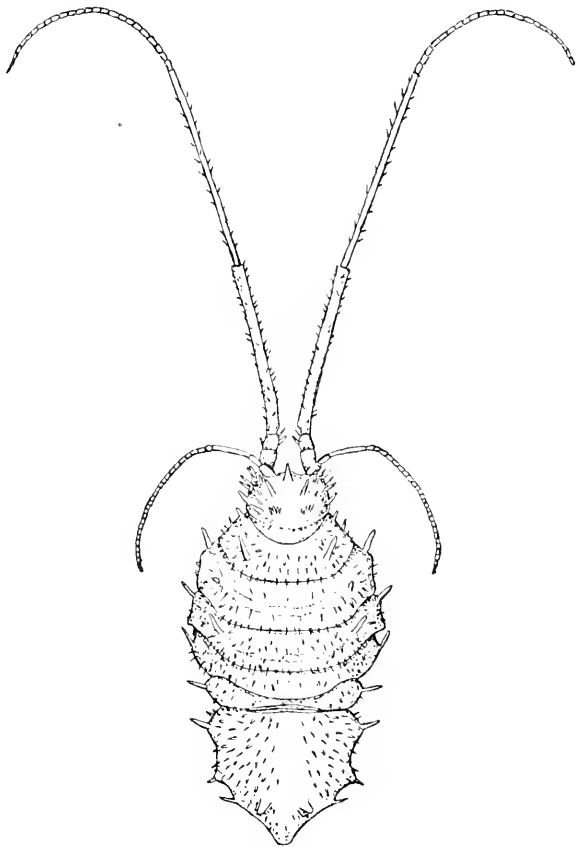
FIG. 541.—MUNNA CECA. \times 6 .
