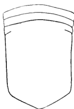
FIG. 391.— Idothea rectilinea . ABDOMEN. \times 63 .
