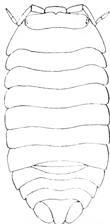
FIG. 707.—ARMADILLIDIUM QUADRIFRONS (LAFETER STOLLER). (x 5).
