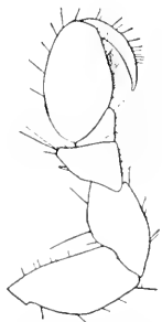
FIG. 489.— ASELLUS TOMALENSIS . LEG OF FIRST PAIR. \times 20 .
