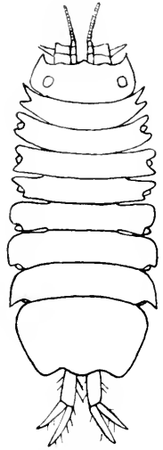
FIG. 520.— IOLELLA EROSTRATA . · 13½.
