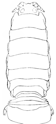
FIG. 219.—MEINERTIA GILBERTI. \times 2\frac{1}{2} .
