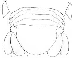
FIG. 197.—ROCINELA PROPODIALIS. ABDOMEN. 21.
