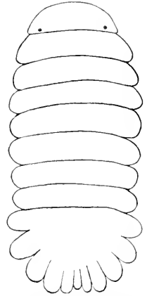
FIG. 609.—PROBOPYRUS BITHYNIS. MALE. 41.
