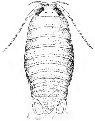
FIG. 123.—EXOCORALLANA MEXICANA. MALE. 6.
