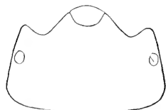
FIG. 533.—JÆROPSIS LOBATA. HEAD. \times 27\frac{1}{2} .
