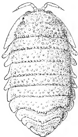
FIG. 700.—PSEUDARMADILLO DOLLI- FUSI. . . 7.
