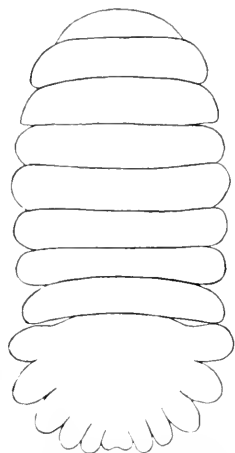
FIG. 611.—PROBOPYRUS BITHYNIS. MALE. × 41.
