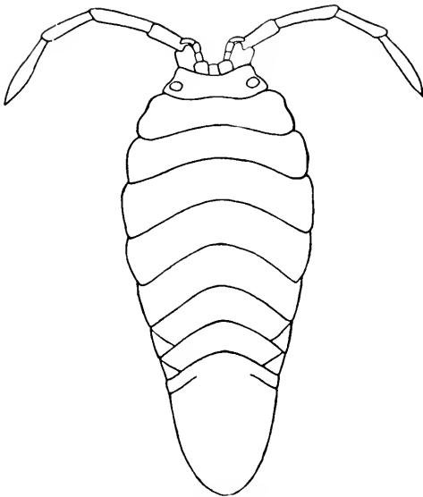
FIG. 415.—EUSYMMERUS ANTENNATUS. — S.
