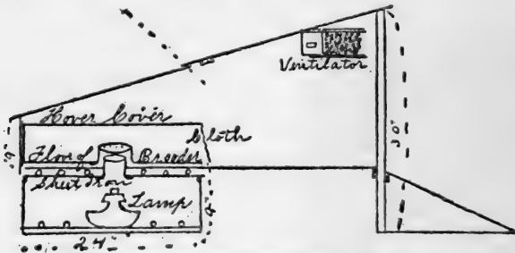
HOMEMADE BROODER. FIG. 15.
