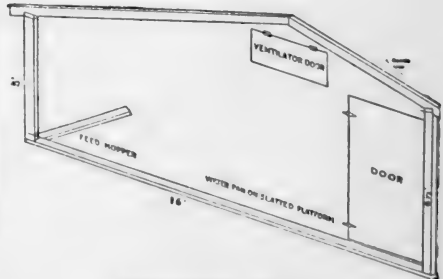
END VIEW. FIG. 27.
