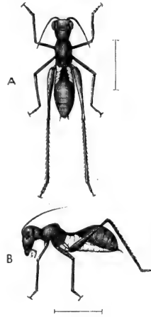
FIG. 199.— Myrmecophana fallax .
