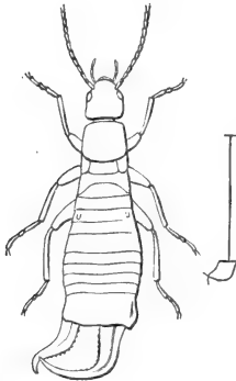
FIG. 113.— Anisolabis tasmanica ♂.
