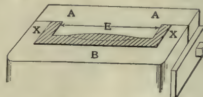
Fig. 2.—Crosshead Babbitting Jig.
