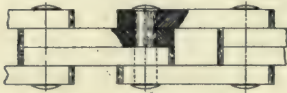
Fig. 1.—Dredge Chain.
