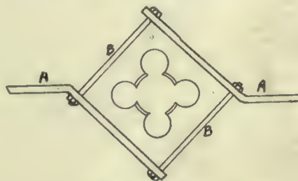
Useful Die Holder.
