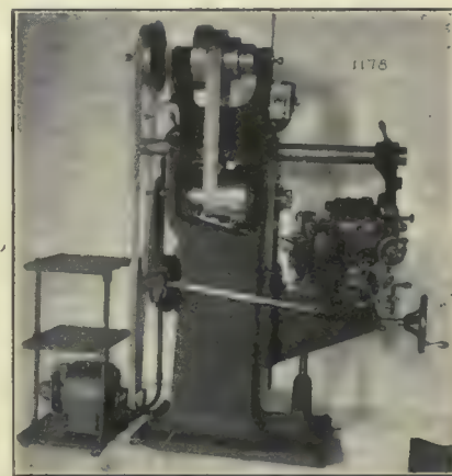
Fig. 2.—No. 1½ Universal Milling Machine Motor Mount.
