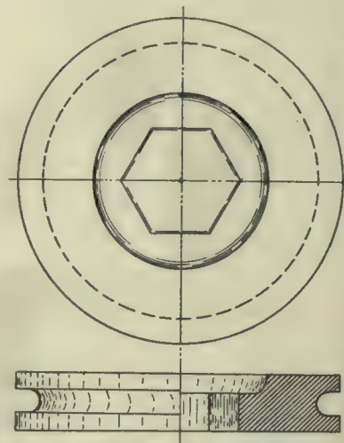
Fig. 7.—Forge Die for Crank Pin Nut.
