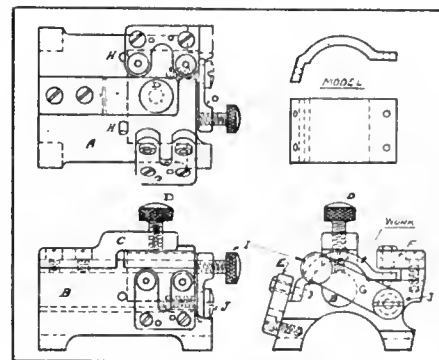
A DRILL JIG.
