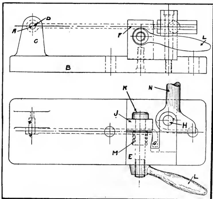
BENDING JIG.
