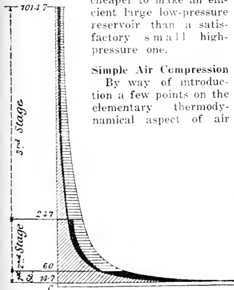
FIG. 1. PV DIAGRAM.
