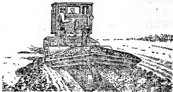
圖11 犂式开溝机 KM—800
