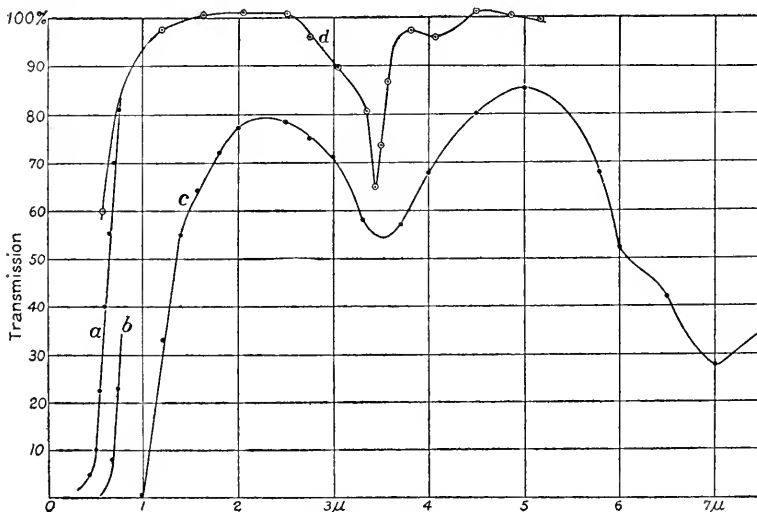
FIG. 31. — Asphaltum.
