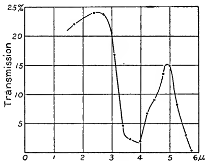
FIG. 27. — Siderite.
