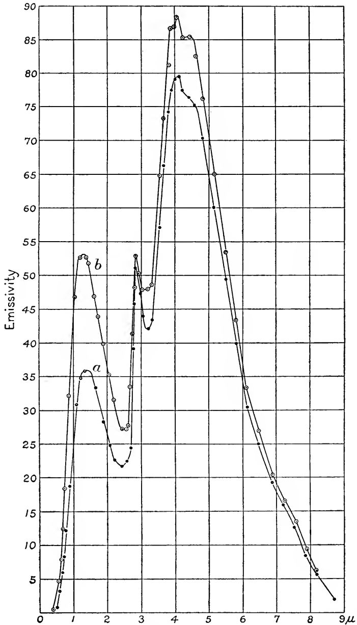
FIG. 74. — Topaz.
