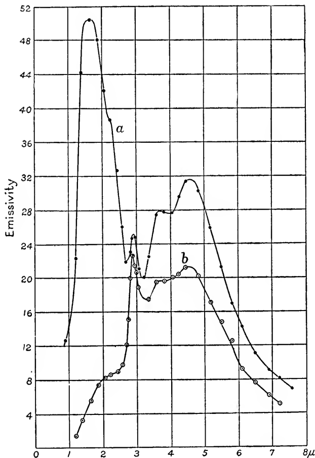
FIG. 68. — Wollastonite.
