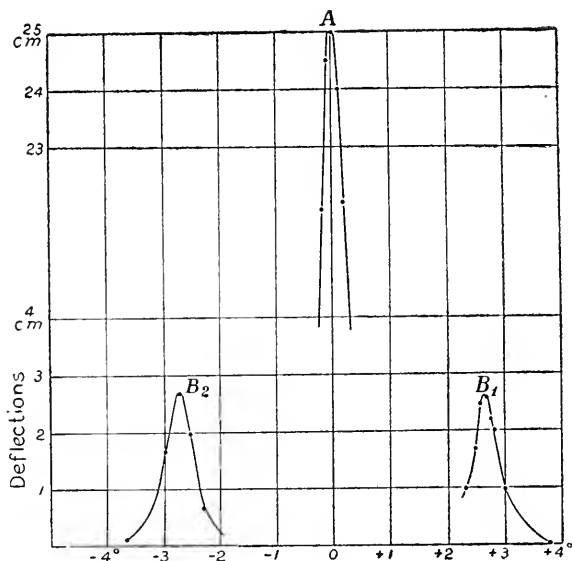
FIG. 23.—Cryolite.
