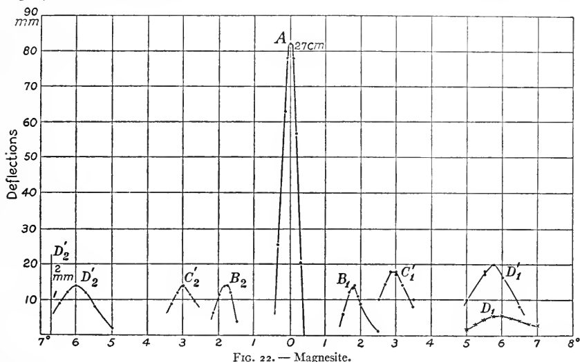
FIG. 22. — Magnesite.
