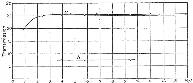
FIG. 25. — Molybdenite.
