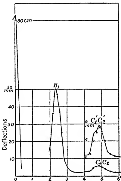
FIG. 20. — Muscovite mica.
