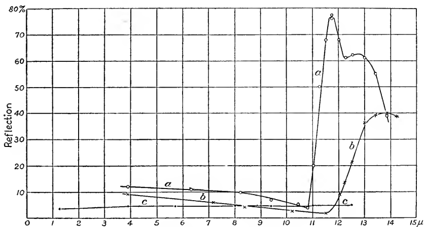
FIG. 9. — Wulfenite ( a ); Rutile ( b ); Zincite.
