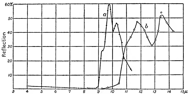
FIG. 10. — Cyanite ( a ); Corundum.
