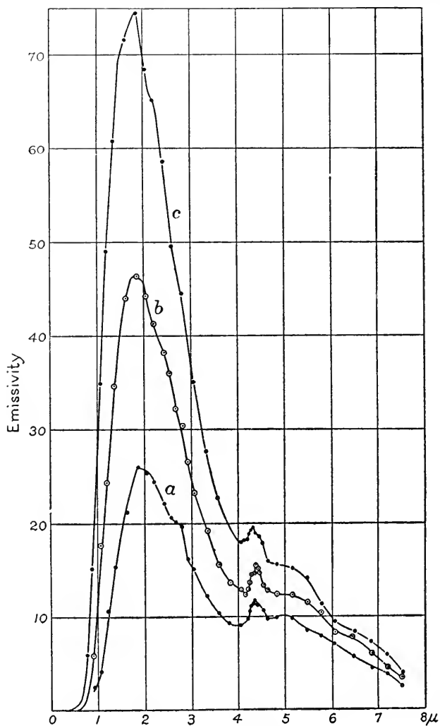
FIG. 78. — Zirconium oxide.
