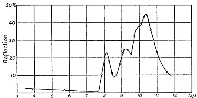
FIG. 11. — Beryl.
