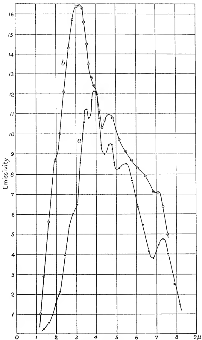
FIG. 02. — Calcite.
