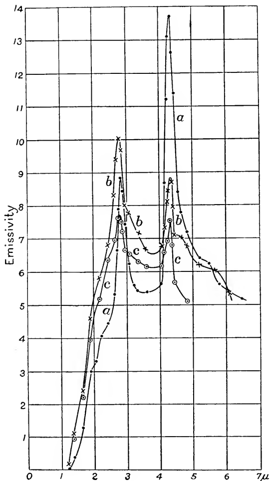
FIG. 79. — Zirconium oxide.
