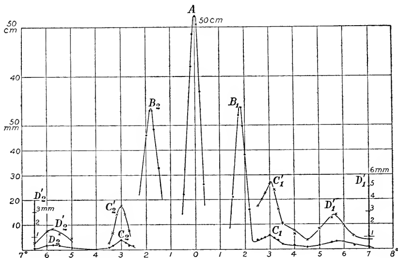
FIG. 21. — Calcite.
