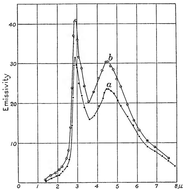
FIG. 75.—Apatite.
