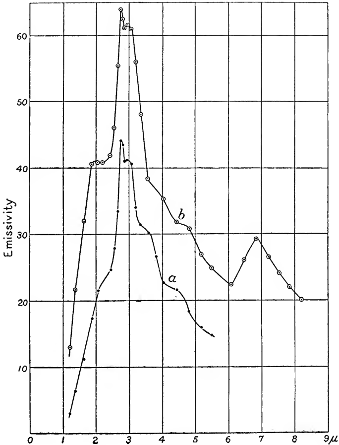
FIG. 83.—Yttrium oxide.
