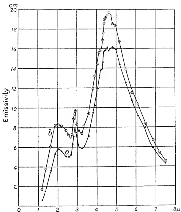
FIG. 72. — Spodumene.
