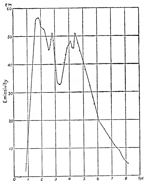
FIG. 69.—Porcelain.
