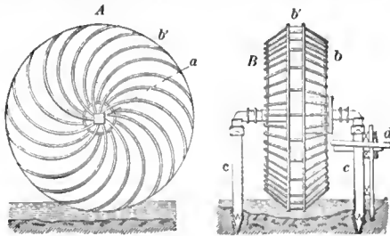
Ferronnet's Tympanum.
