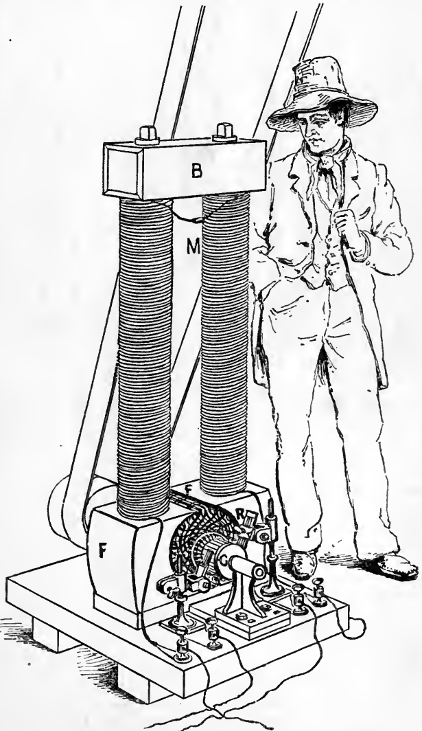
FIG. 10. FARADIC GENERATOR.
