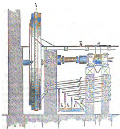
Fig. 2.—Ore Mill:
