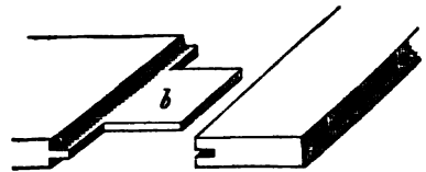
Mortise and Tenon : a, mortise; b, tenon.
