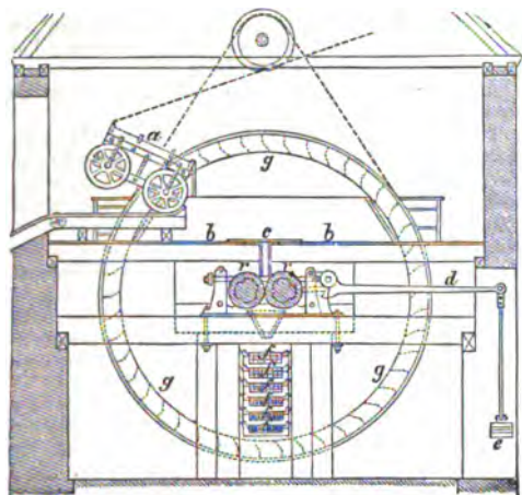
Fig. 1.—Ore Mill:
