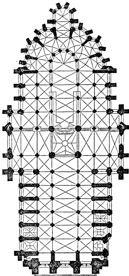
Fig. 12.—Amiens Cathedral.
