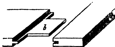
Mortise and Tenon : a, mortise; b, tenon.
