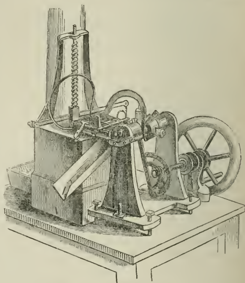
Fig. 1.—Type-casting Machine.
