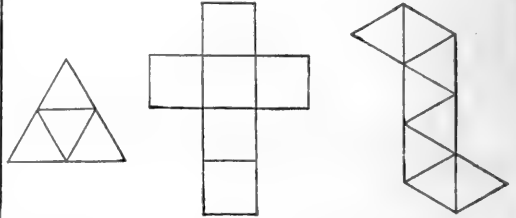
Tetrahedron.
