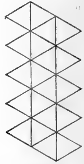
Icosahedron.
