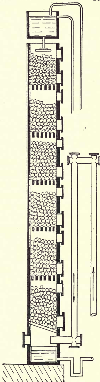
FIG. 26. MITSCHERLICH ACID TOWER
