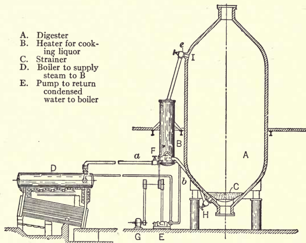
FIG. 8. MORTERUD DIGESTER
