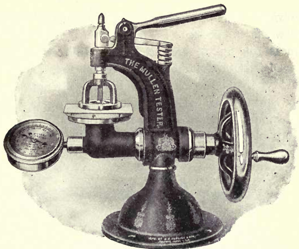
FIG. 51. MULLEN TESTER
