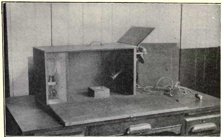
FIG. 49. INGERSOLL GLARIMETER
