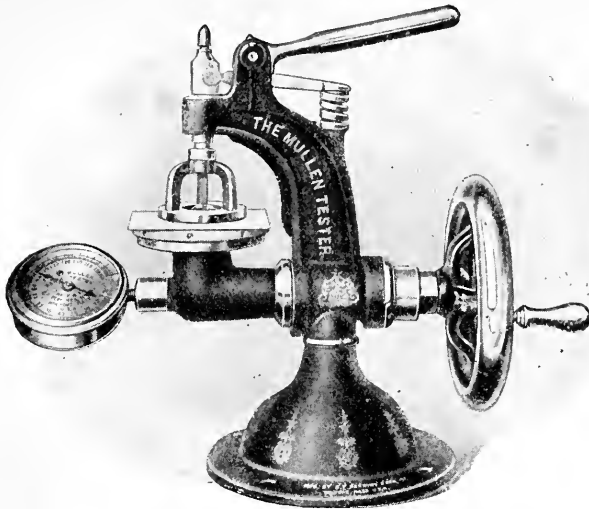
FIG. 51. MULLEN TESTER
