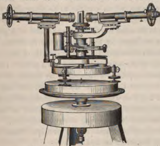
FIG. 34.—Ångström's spectrometer.
