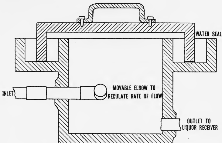
FIG. 32.—Water Box.
