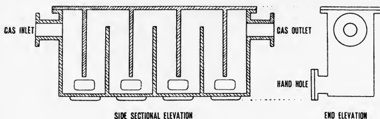
FIG. 45.—Dust Separator.
