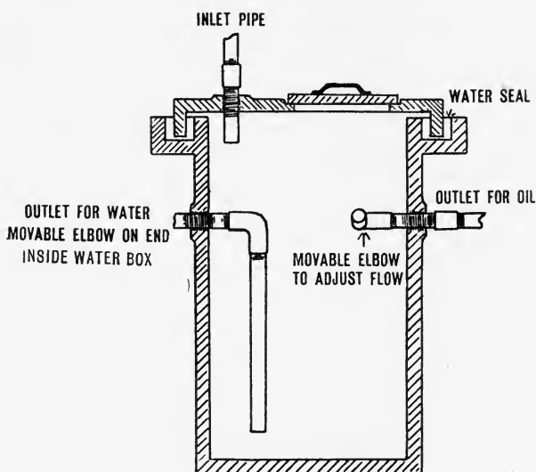
FIG. 31.—Dividing Box.
