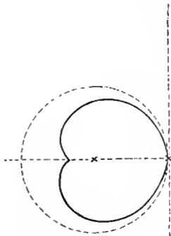
Fig. 8. a = 1 .
