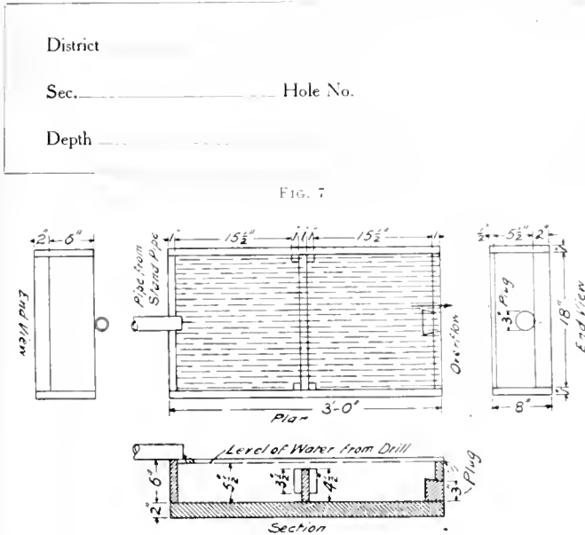
FIG. 8. SLUDGE BOX
