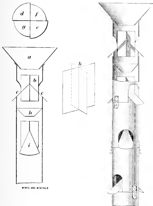
FIG. 1. PIPE SAMPLER
