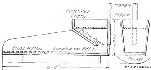
FIG. 1. THE ROCKER
