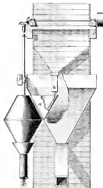
FIG. 3. VEZIN SAMPLER
