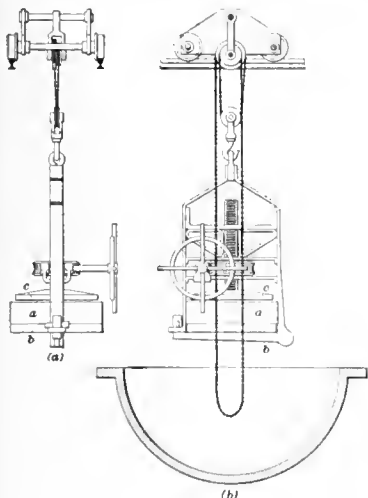
FIG. 4. HOWARD PRESS
