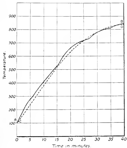
FIG. 2. GALENA-SILICA ROAST
