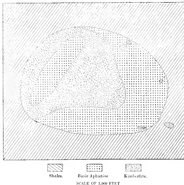
HORIZONTAL SECTION OF PIPE AT VOORSPOED MINE
