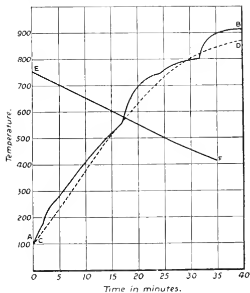
FIG. 1. GALENA-LIME ROAST
