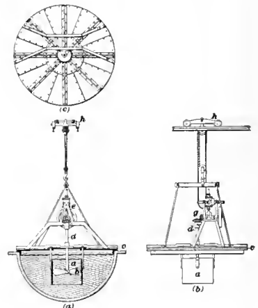
FIG. 3. HOWARD STIRRER
