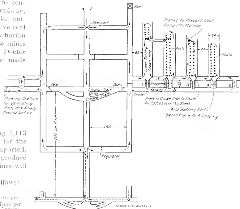
FIG. 1. PLAN OF COMO MINE
