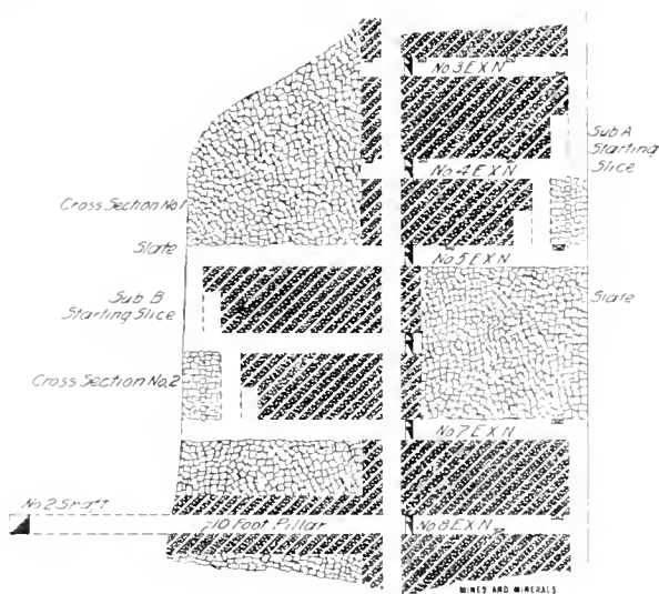
FIG. 3. PLAN.
