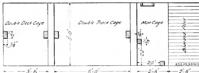
FIG. 2. PLAN OF EL PASO SHAFT
