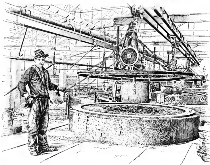
FIG. 2. DROSSING KETTLE
