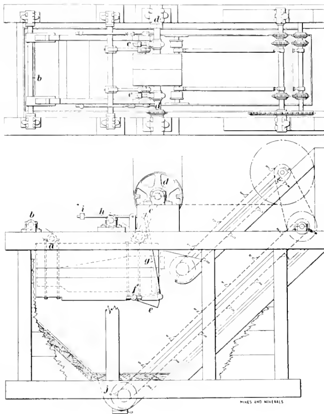
B. & K. COAL JIG
