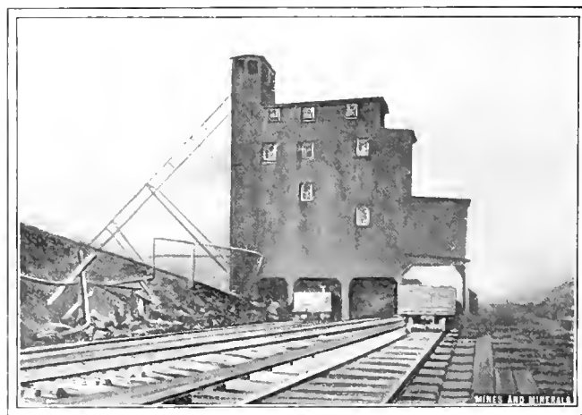
FIG. 5. SHIAWASSEE TIPPLE
