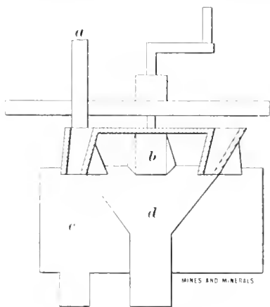
FIG. 4. BRIDGEMAN SAMPLER
