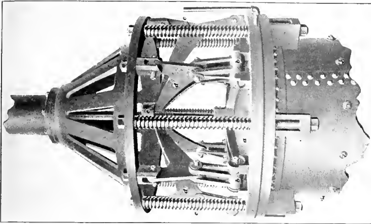
FIG. 3. DISCHARGE DOOR MECHANISM
