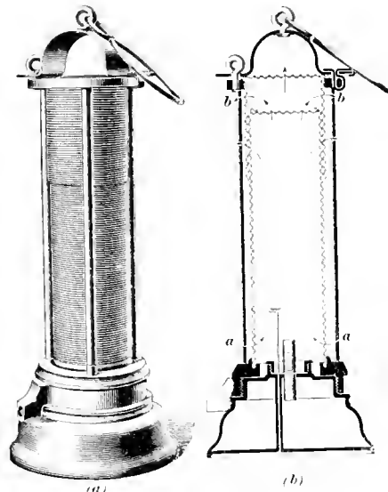
FIG. 1. DAVY LAMP
