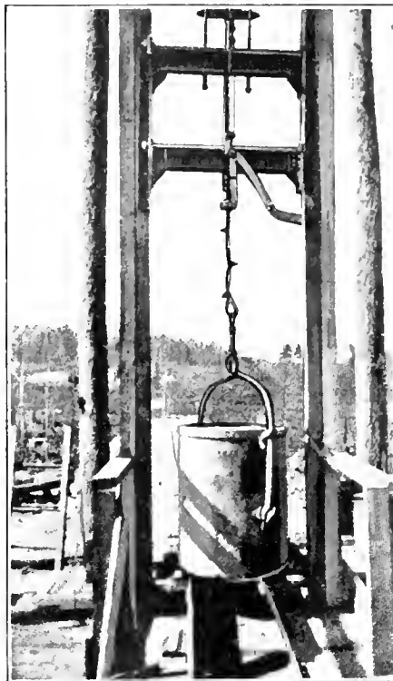
FIG. 1. MORIN CROSSHEAD
