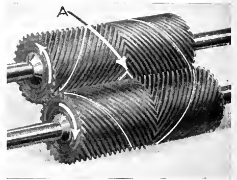
FIG. 9. THE ROTORS
