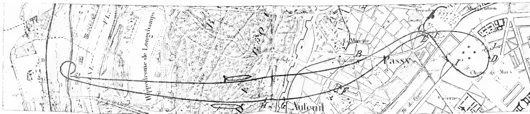
Tracé sur la Carte du Service géographique de l'Armée au \frac{1}{25000} de la trajectoire horizontale de l'aérostat de M. Santos-Dumont, dans l'expérience du 19 octobre 1901
