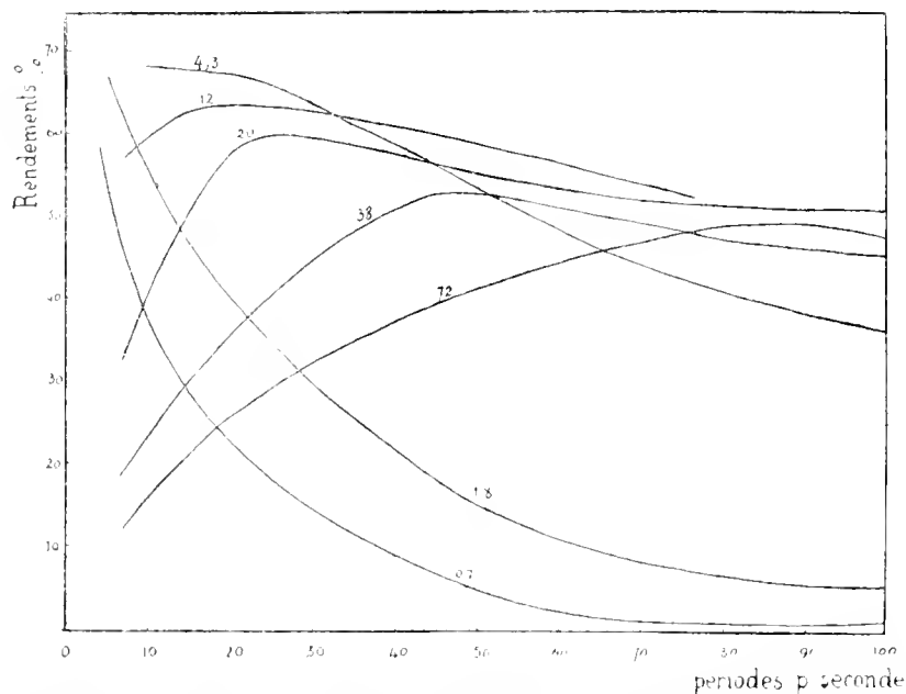
Électrolyse par courant alternatif. Variation du rendement en fonction de la fréquence pour diverses densités de courant.
