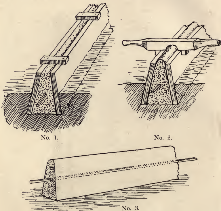
Fig. 43.—GARDEN KERB.
