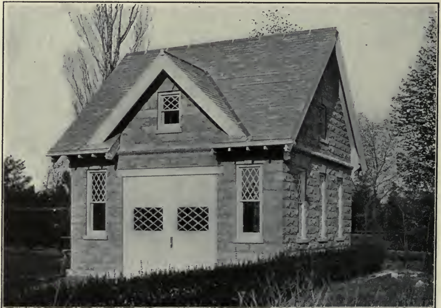
Concrete Block Garage, Paterson, N. J.
