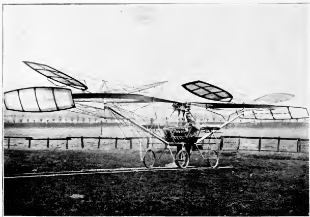
CORNU'S HÉLICOPTÈRE
