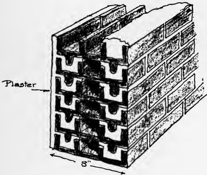
FISKLOCK BRICK
