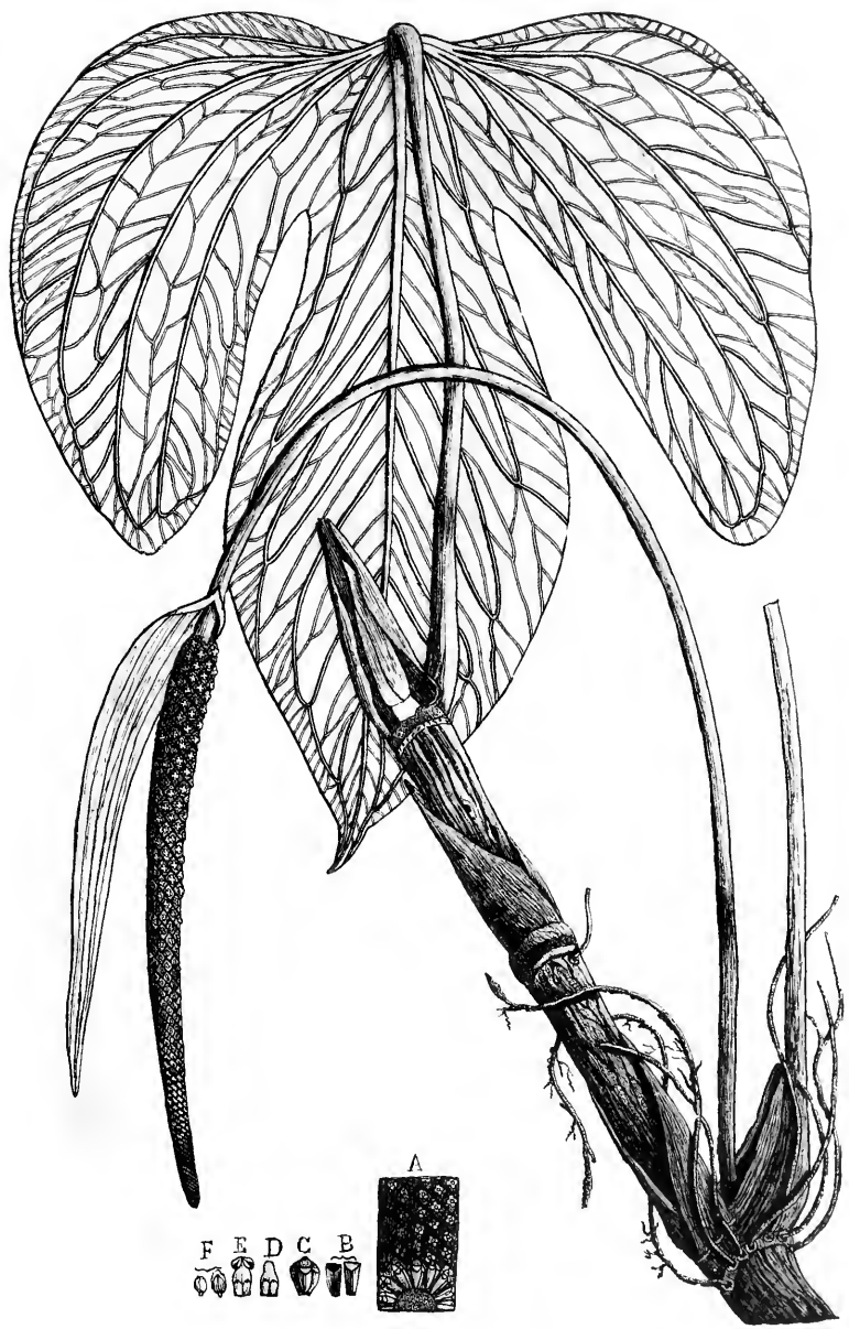
A TRUNCICOLUM Engler.
