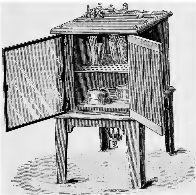
FIG. 10.—INCUBATOR.
