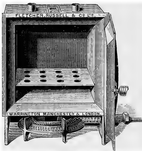
FIG. 6.—HOT-AIR STERILIZER.
