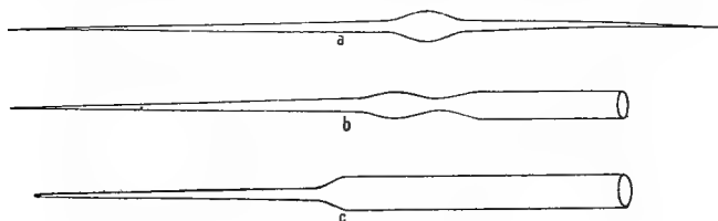
FIG. 14.—PIPETTES.
