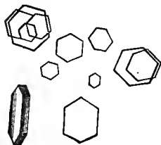
FIG. 10.—CYSTIN.
