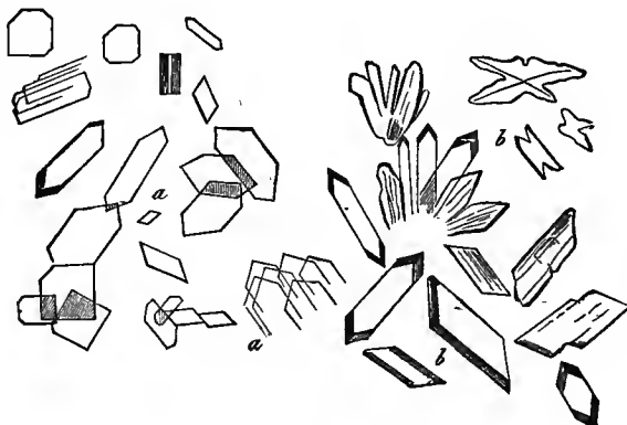
Fig. 14.— a , Urea Nitrate; b , Urea Oxalate.
