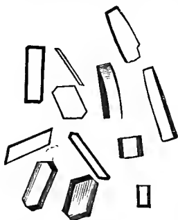
Fig. 6.—Glycocoll.
