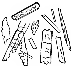
FIG. 28.—Benzoic acid.
