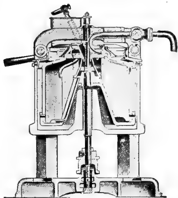
FIG. 48.—The Reid separator.
