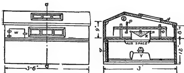
FIG. 85—DR. WOODS' BROODER
