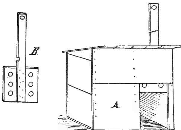
FIG. 57—CONVENIENT BOX COOP
