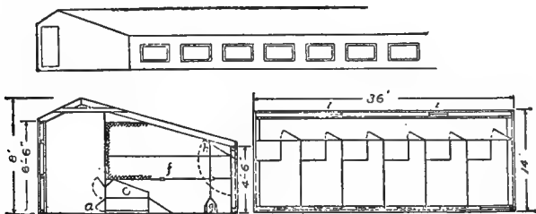
FIG. 72— PLAN OF SIMPLE BROODER HOUSE
