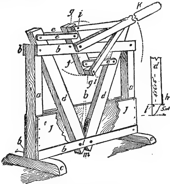
FIG. 52—GRIT CRUSHER
