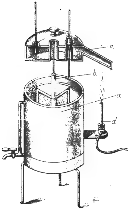
FIG. 53.—Slow steriliser for blood serum.
