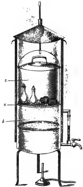
FIG. 14.--"Steam steriliser."
