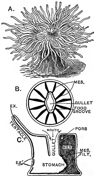
Fig. 290.—Sea-Anemone
