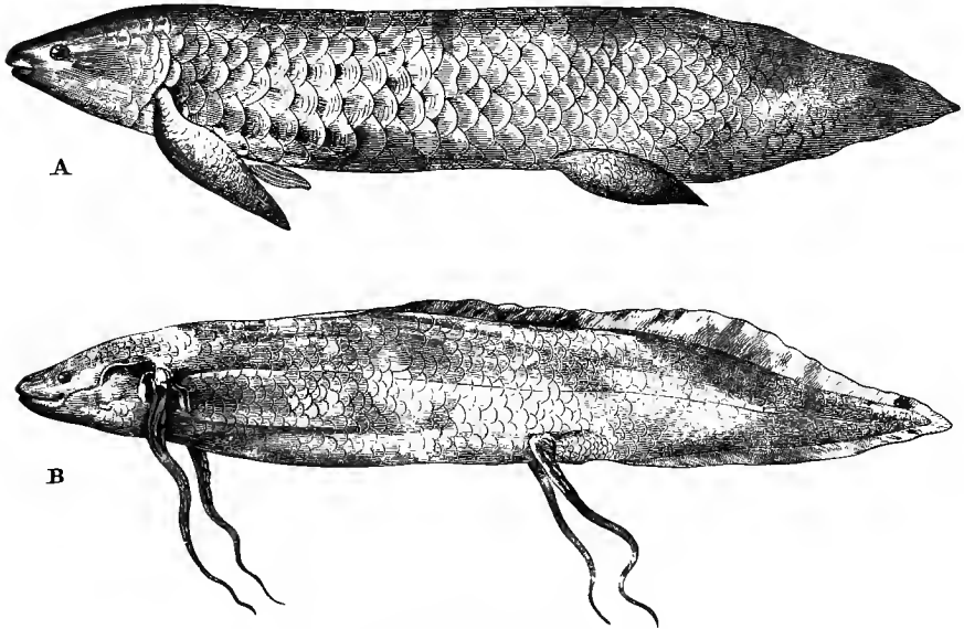
Fig. 161.—Dipnoi
