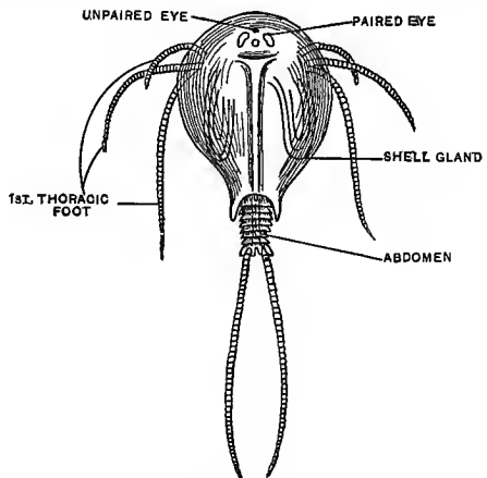
Fig. 261.— Apus
