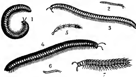
Fig. 245.—British Millipedes
