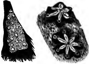
Fig. 174.— Botryllus
