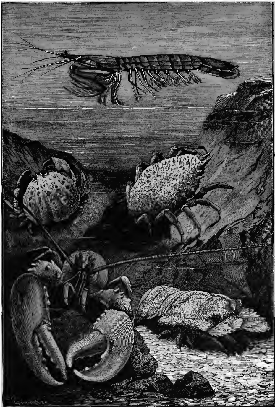
Fig. 230.—Mediterranean Crustacea
