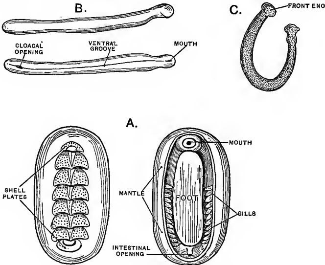
Fig. 200.—Proto-molluscs
