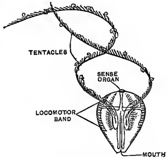
Fig. 297.— Cydidippe
