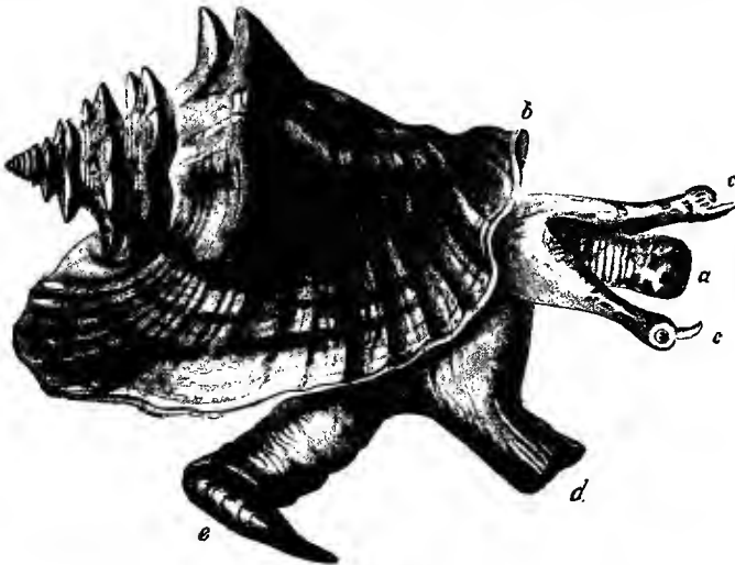
Fig. 185.— Strombus
