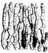
Fig. 5.— Syringopora retiformis . Silurian.
