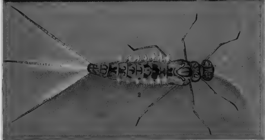
Callibaetis skokiana
