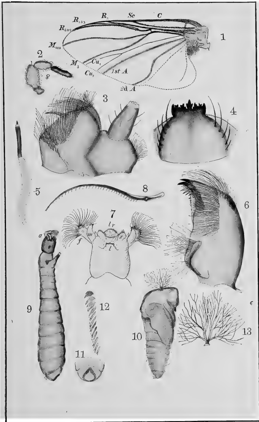
hirtipes
