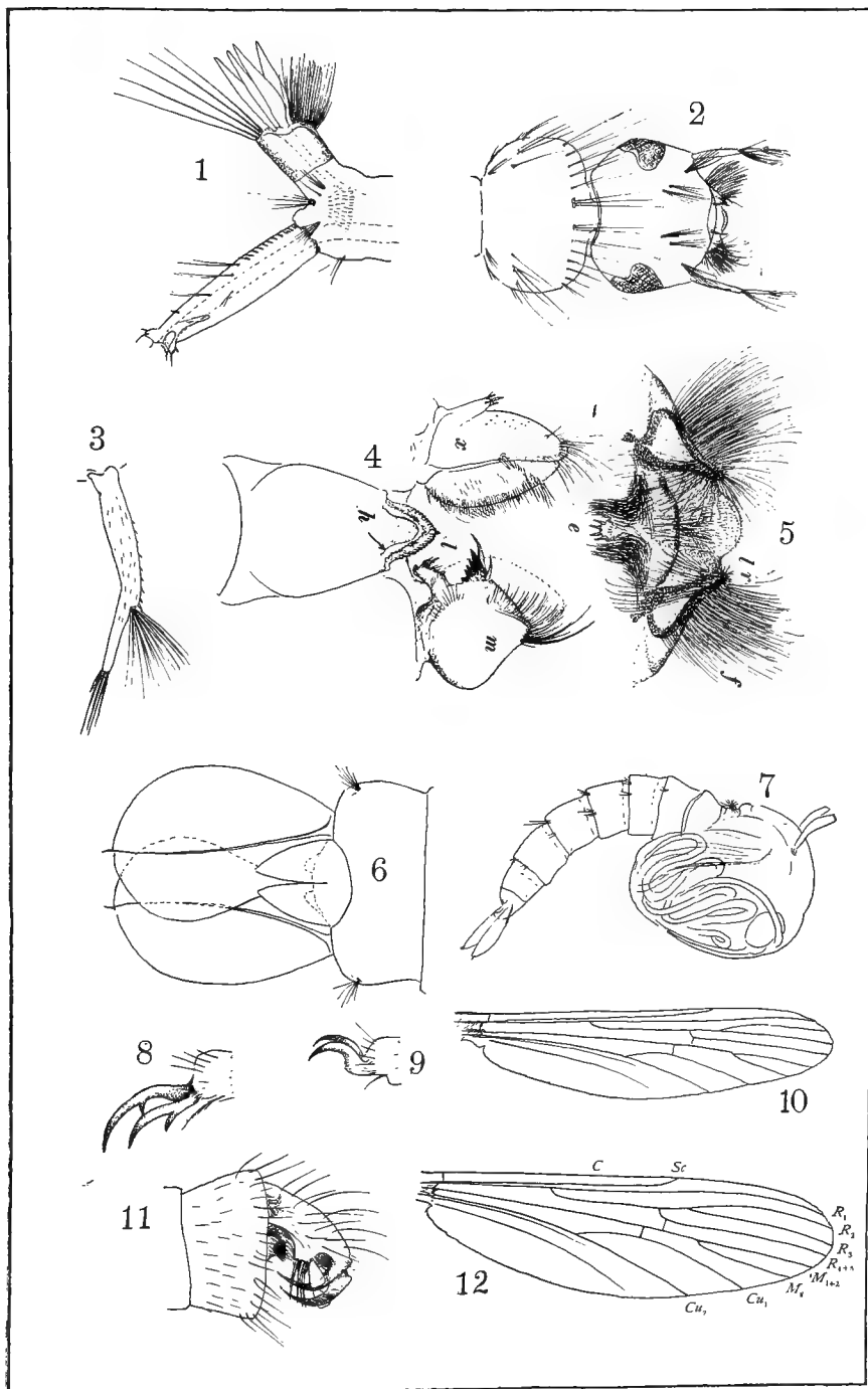
Culex pipiens
