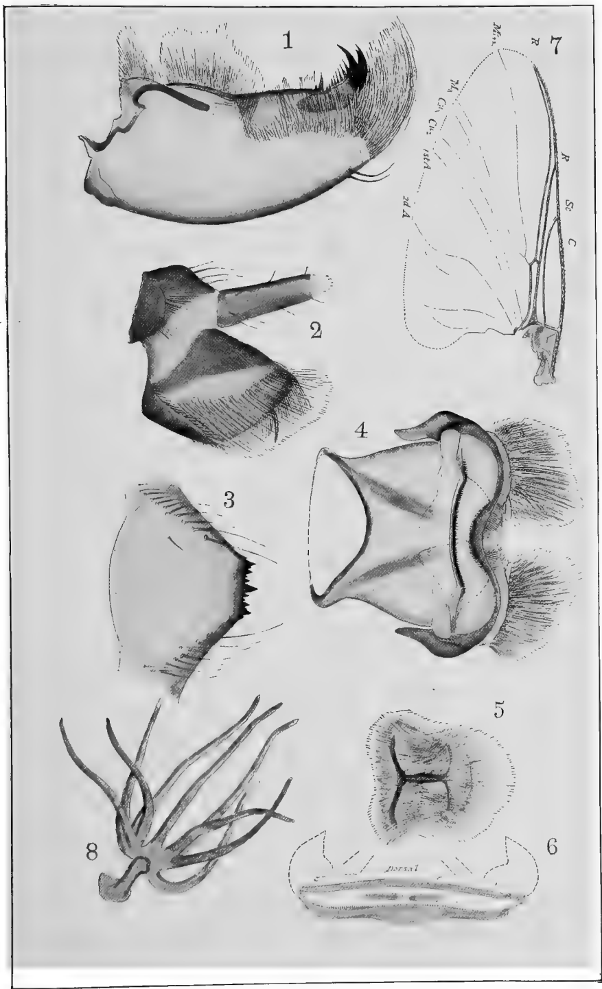
pictipes
