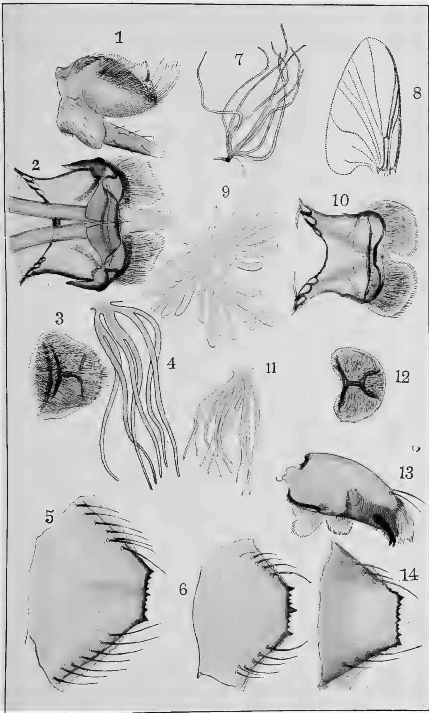
Stimulium venustum
