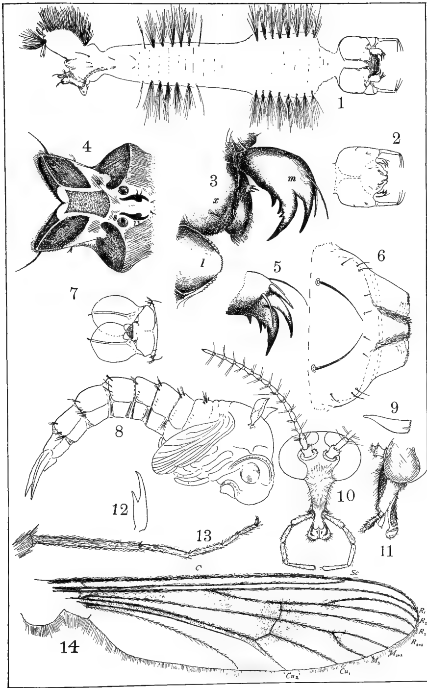
americana
