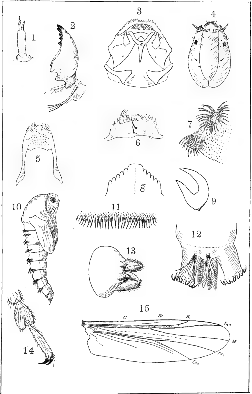
Thalassomyia obscura
