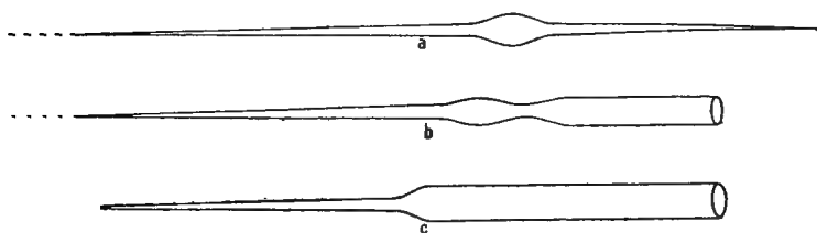
FIG. 12.—Pipettes.
