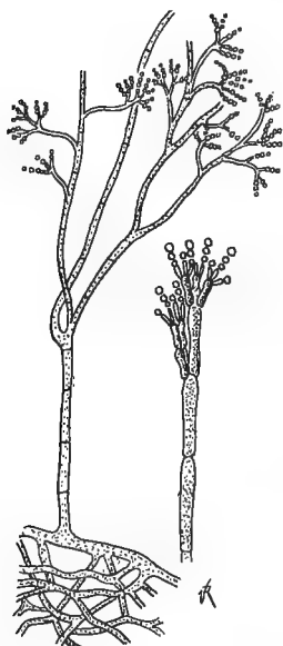
FIG. 16.— Penicillium .
