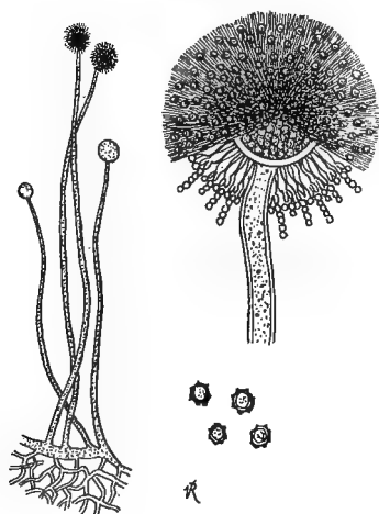
FIG. 17.— Aspergillus .
