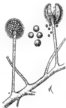
FIG. 19.— Mucor .
