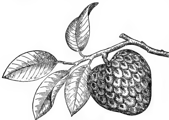
425. Cherimoya.
