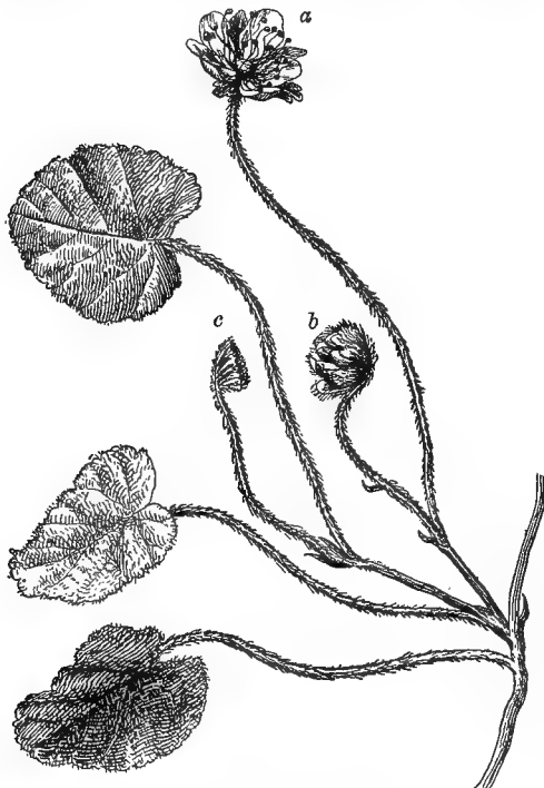
673. Dalibarda repens .
