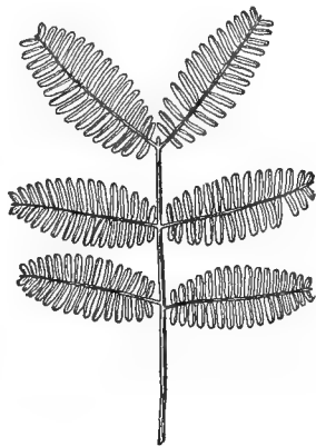
10. Acacia Arabica.
