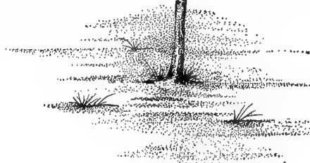
631. Cyathea meridensis .
