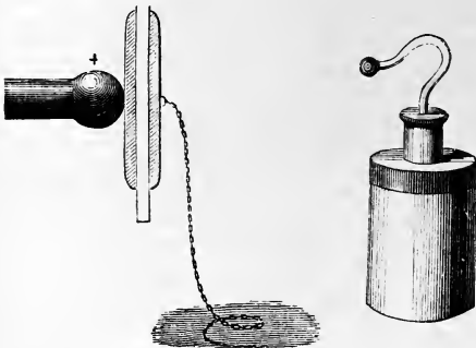
FIG. 15.—Condenser.
