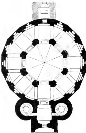
Abb. 10 Grundriß des Münsters zu Aachen
