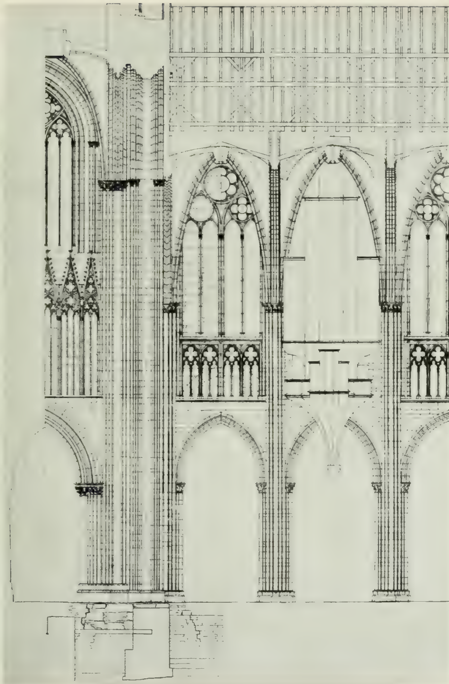
TEIL DES LÄNGSSCHNITTS - TURMJOCH UND LANGHAUSJOCH
