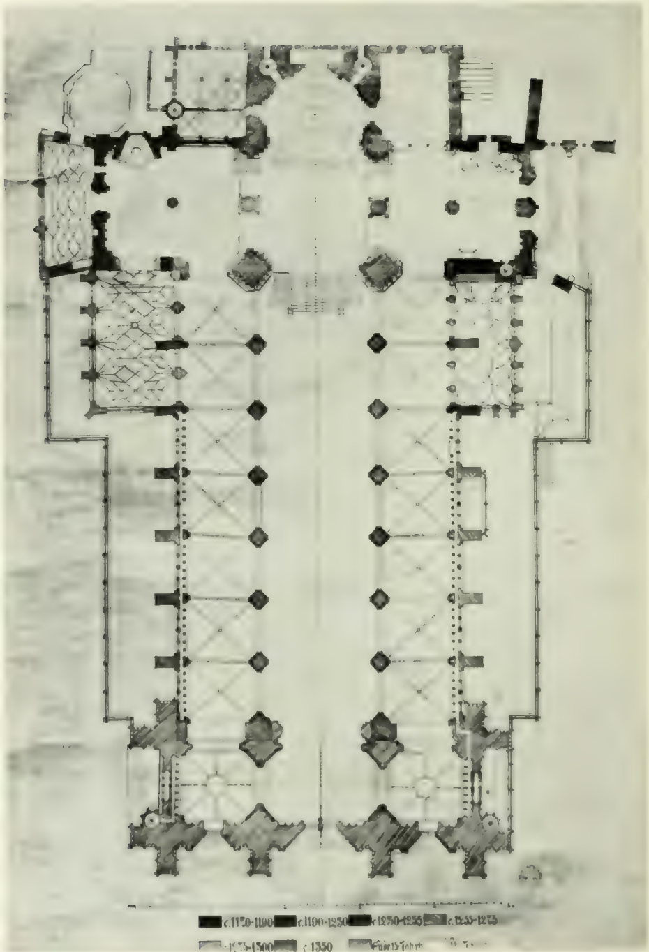
GRUNDRISS - GEGENWÄRTIGER ZUSTAND
