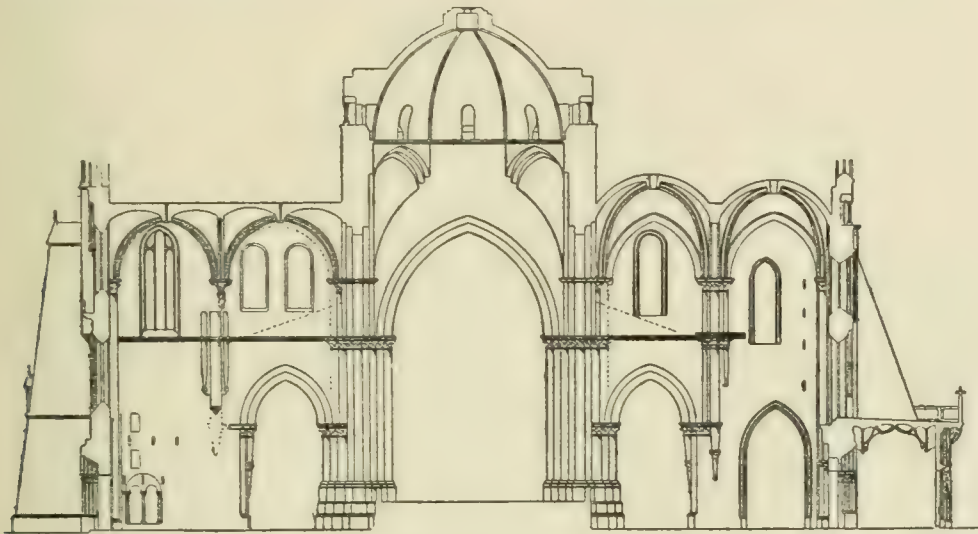
ABB. A: SCHNITT DURCH QUERHAUS UND VIERUNG (GEGEN WESTEN).
