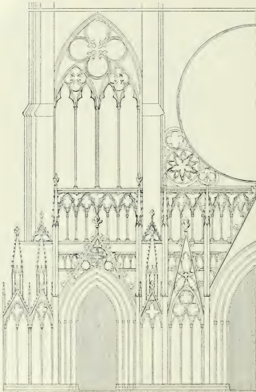
ENTWURF FÜR DIE WESTFASADE. RISS A
