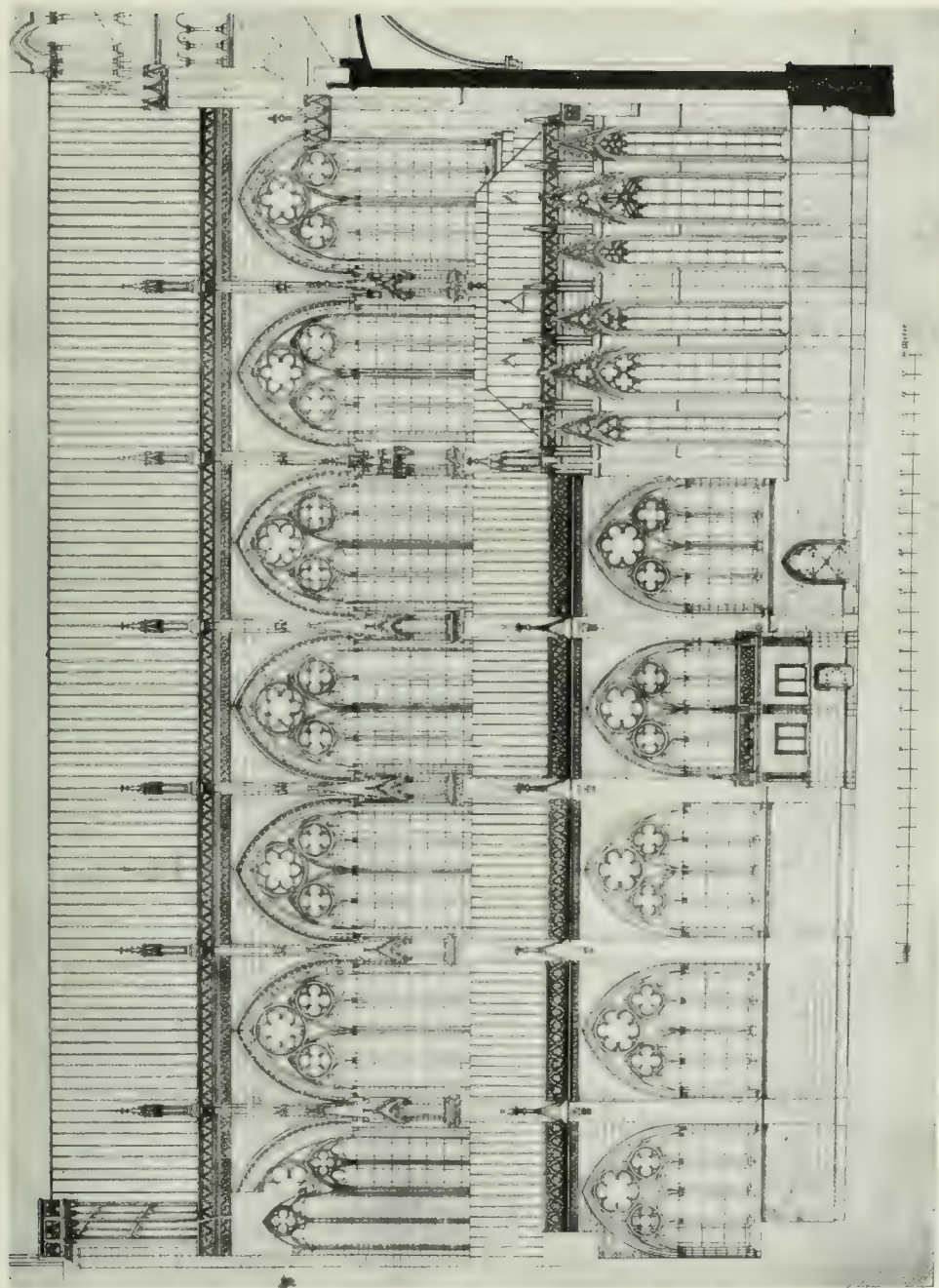
AUFRISS DES LANGHAUSES - SUDSEITE.
