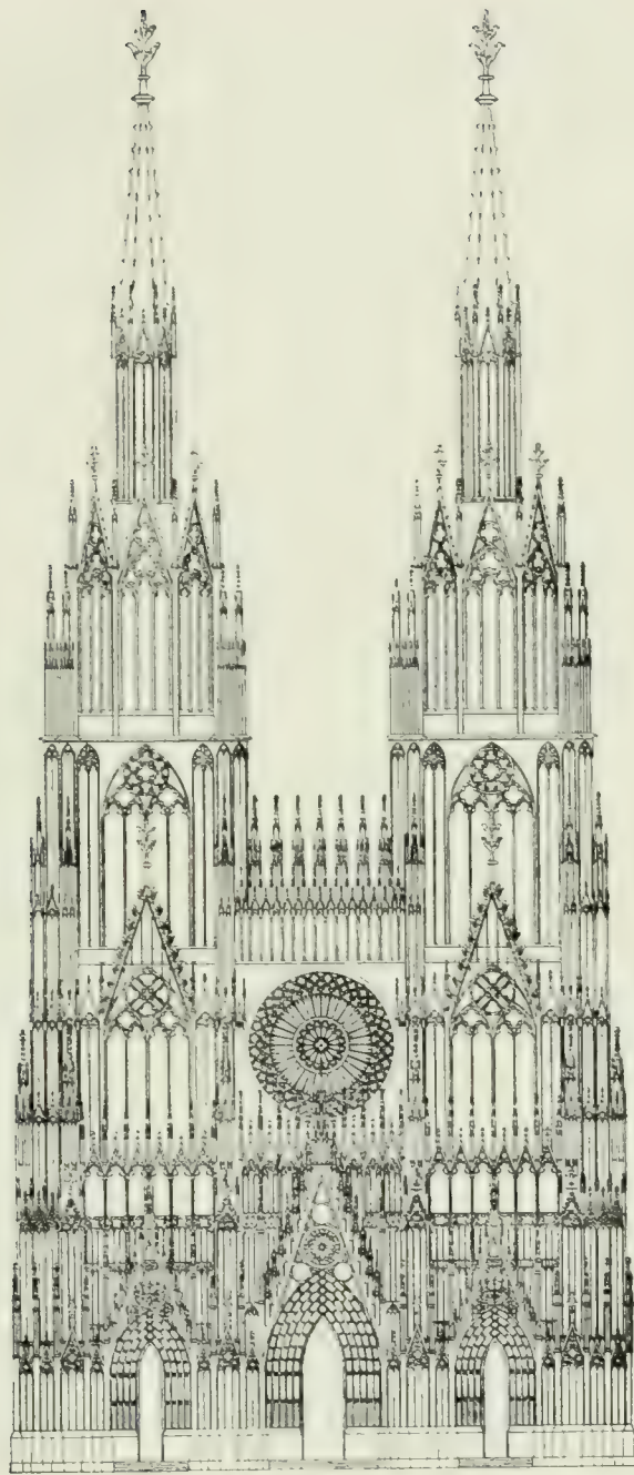
ENTWURF FÜR DIE WESTFASSADE - RISS B
