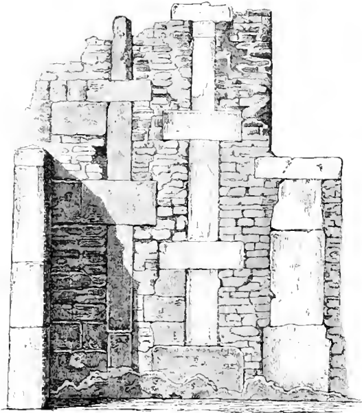
1517 Mauer aus Kalksteinfachwerk.
