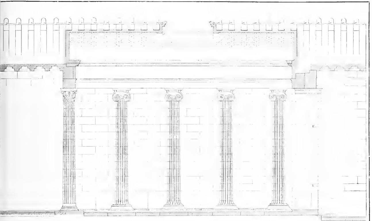
1464 Langendurchschnitt der Tempelcella. (Zu Seite 1320.)
