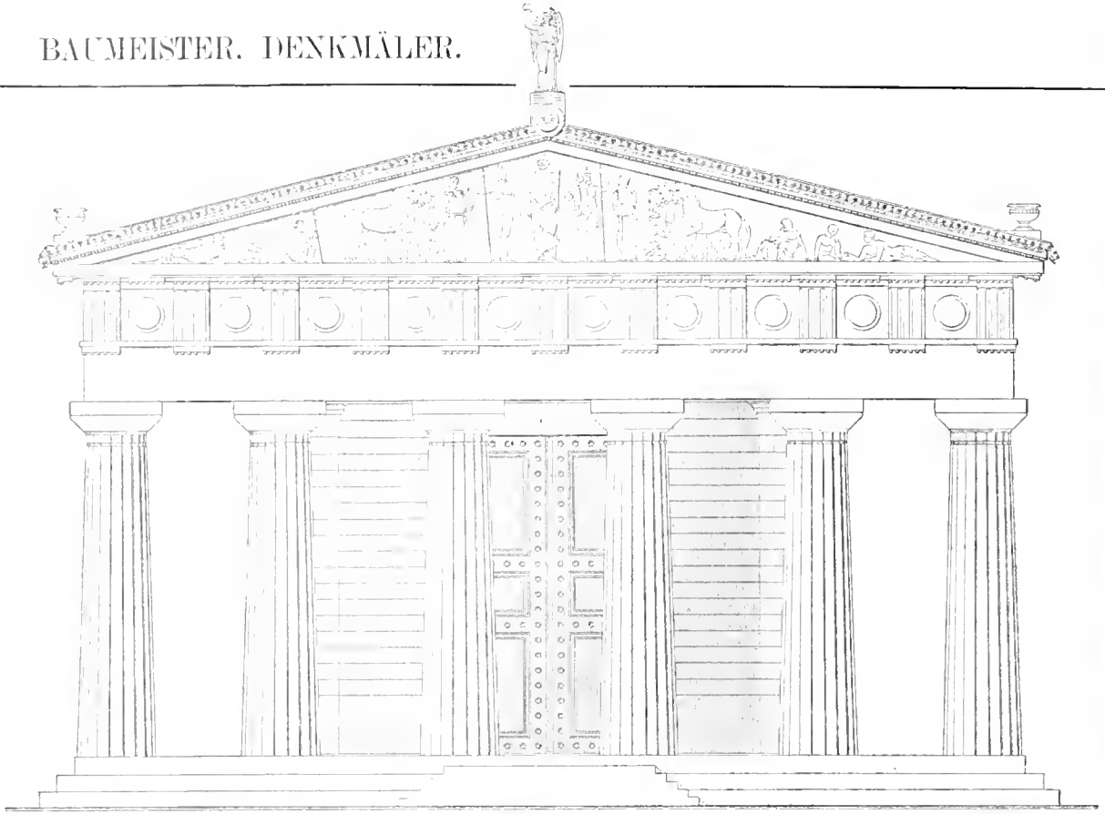
1270 Anfrifs der Ostseite des Zeustempels (Restauration Curtius-Griffither).
