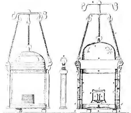
889 Laternen.
