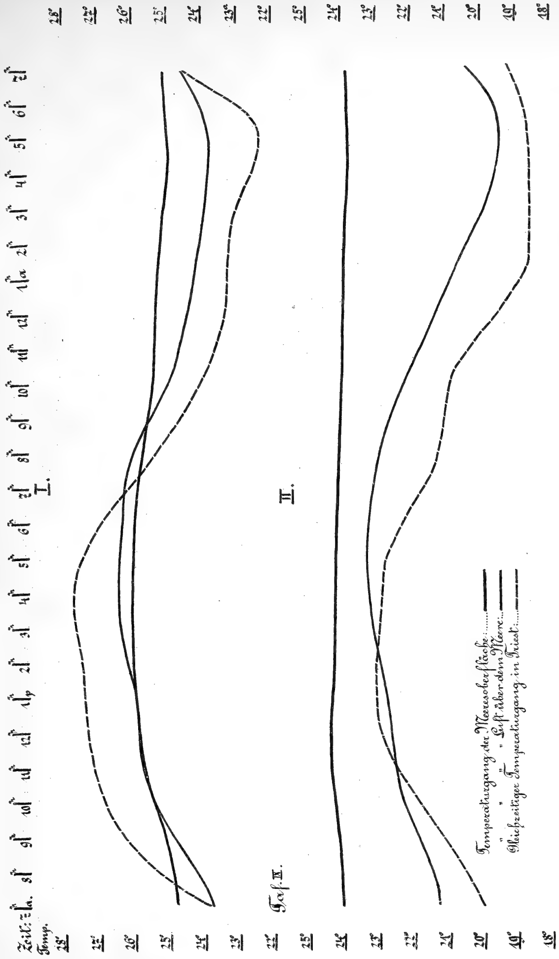
Tafel III. Die Beziehung zwischen Luft- und Wassertemperatur I. an heißen, II. an kühlen Tagen.
