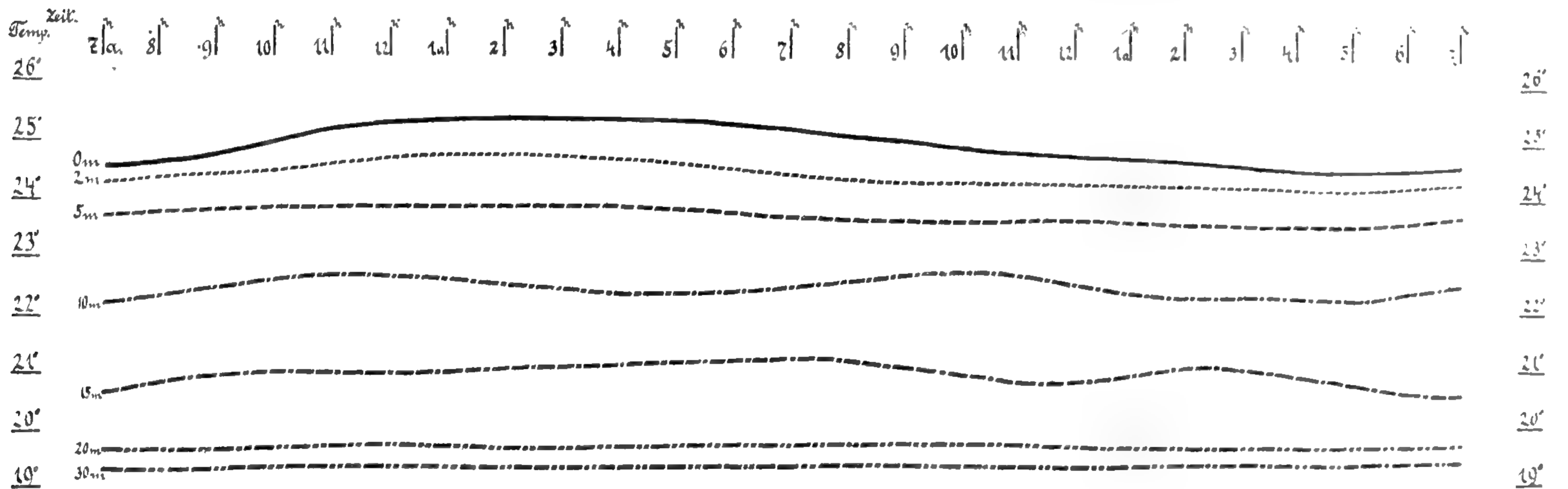
Taf. III. Der tägliche Temperaturgang bis 30m Tiefe (Sommer)
