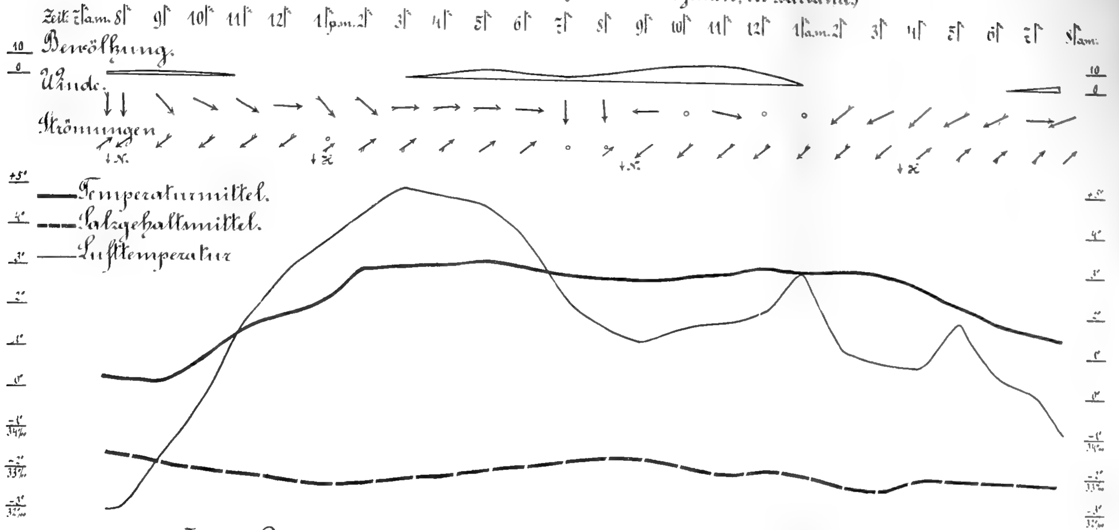
Taf. III. Der tägliche Temperaturgang bis 30m Tiefe (Sommer)
